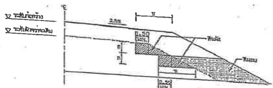
รูปที่ห้า การก่อสร้างลาดชันข้างถนนถมดิน
