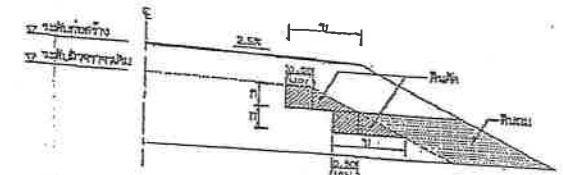
รูปตัดจากถาดสร้างลาดคันทางบนถนนเดิม งานตัด โยธา ฐานคันดิน, งานตัดคันดิน, งานเสริมคันดิน และงานประชิดคัน
