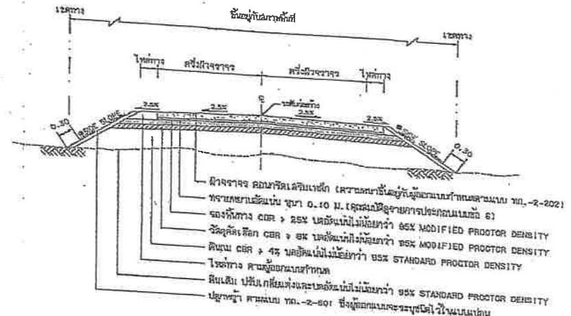
รูปที่สี่ แสดงโครงสร้างถนนลาดชัน เติมน้ำแข็ง และคลุมทับผิวจราจร
